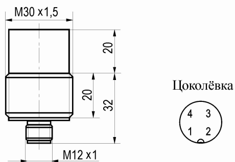
Габаритный чертеж
